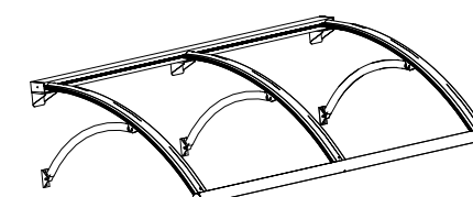
2 specchi - 3 supporti
