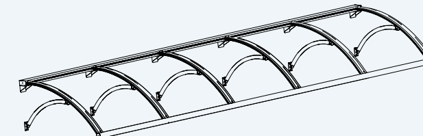
5 specchi - 6 supporti
